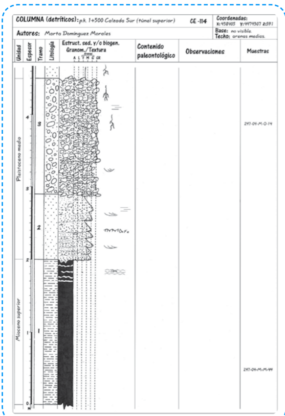
Columna estratigráfica
